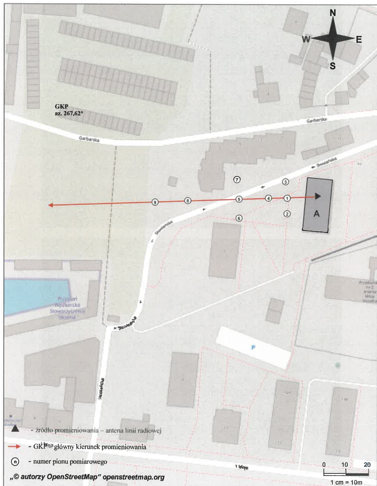
Rys. 1. Usytuowanie punktów i pionów pomiarowych w otoczeniu instalacji radiokomunikacyjnej Stacja Netia GRYOB018-GRYOM00007 Gryfino, ul. Słowiańska 4
