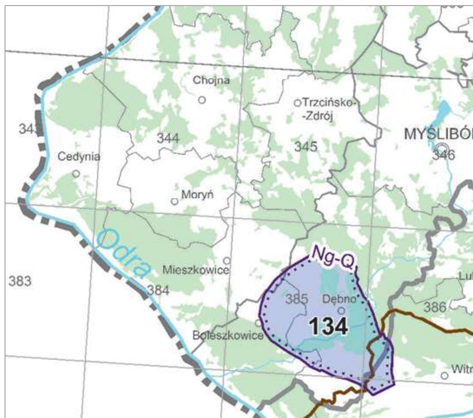
Rysunek 12. Lokalizacja GZWP nr 134 – Zbiornik Dębno Źródło: https://mapy.geoportal.gov.pl/
