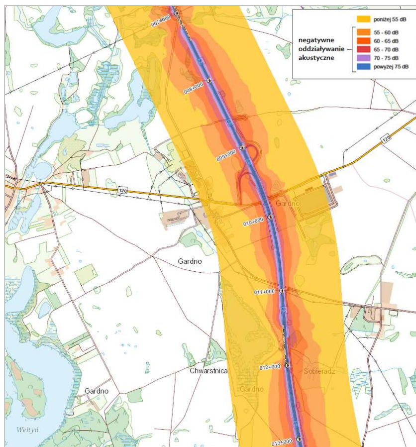
Rysunek 2. Mapa akustyczna dla drogi ekspresowej S3 w rejonie m. Gardno (emisja hałasu – wskaźnik L_{DWN} )
